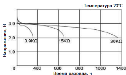
Разряд при различных нагрузках
