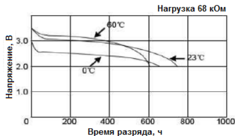
Разряд при различных температурах
