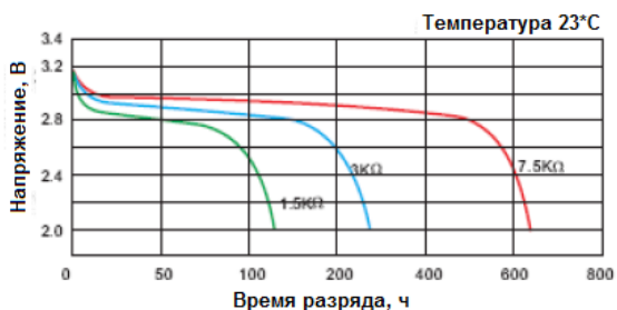
Разряд при различных нагрузках
