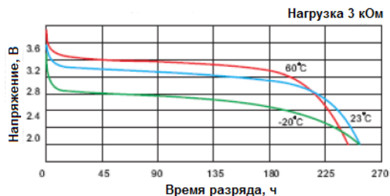
Разряд при различных температурах
