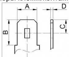
Размеры клемм/контактов F2
